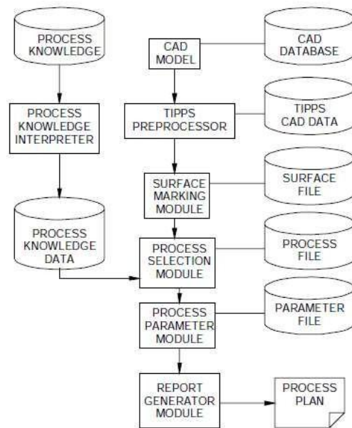
Fig. 17 TIPPS
